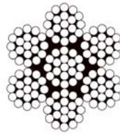
7X19
